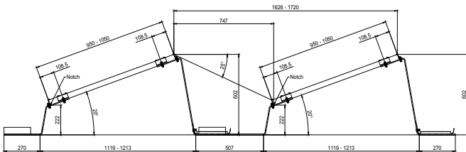
LEICHTmount Freiland S mit einer Modulneigung von 20°
