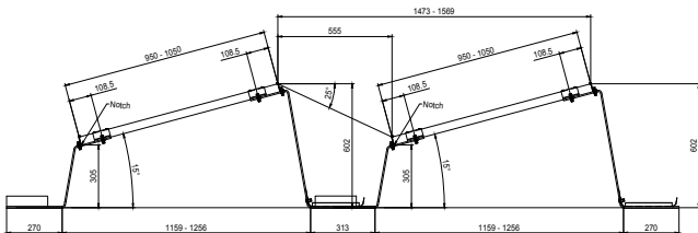
LEICHTmount Freiland S mit einer Modulneigung von 15°
