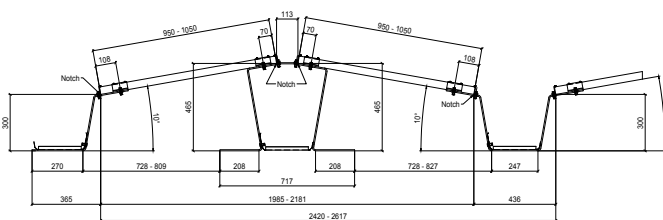
LEICHTmount Freiland EW mit einer Modulneigung von 10°
